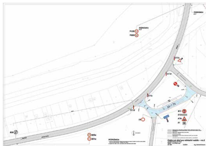
Návrh kontrolního stanoviště u měnínské bažantnice
